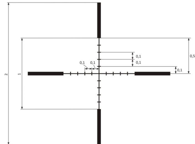
Рисунок 30 – Прицельная сетка (размер в м/100м дистанции)
