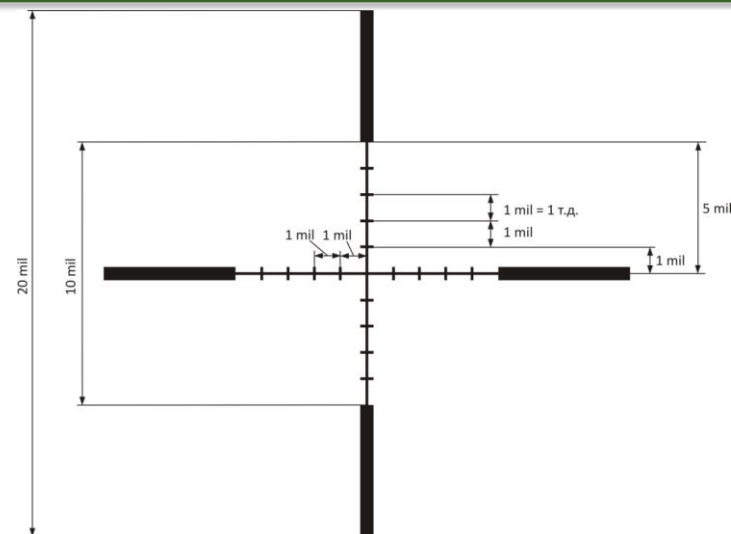
Рисунок 29 – Прицельная сетка (размер в миллирадианах или в т.д.)
